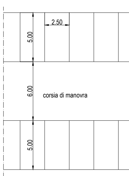
DISPOSIZIONE A PETTINE
